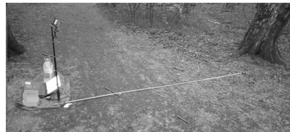
Фотография экспериментальной установки с одним ведомым модулем
